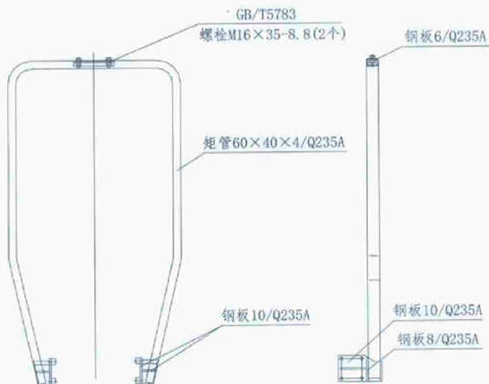
图4-3 防翻架结构图
