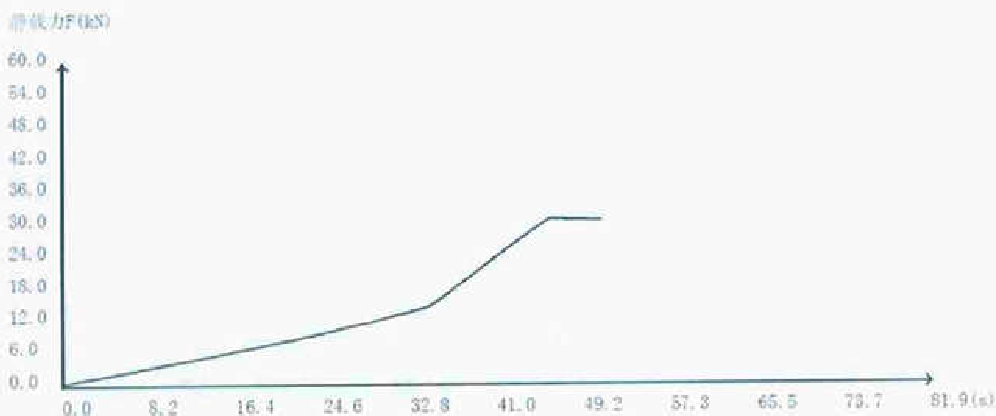
图9 前压垮试验时载荷—时间曲线图
