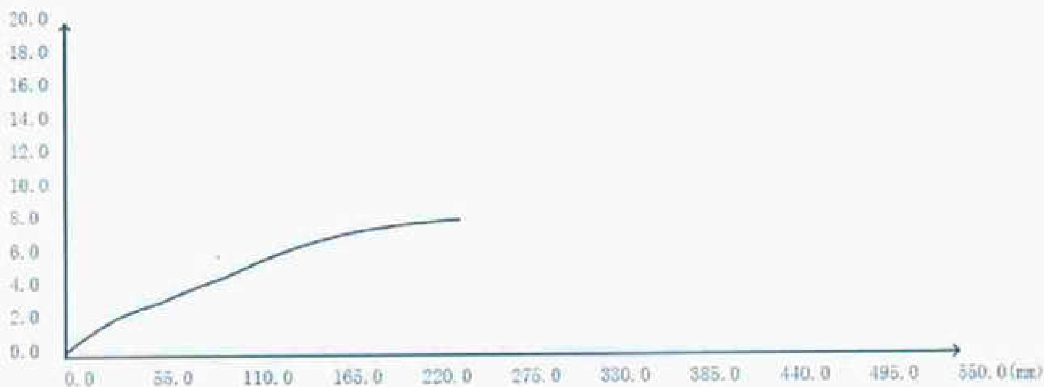
图7 前加载试验时载荷—位移曲线图
