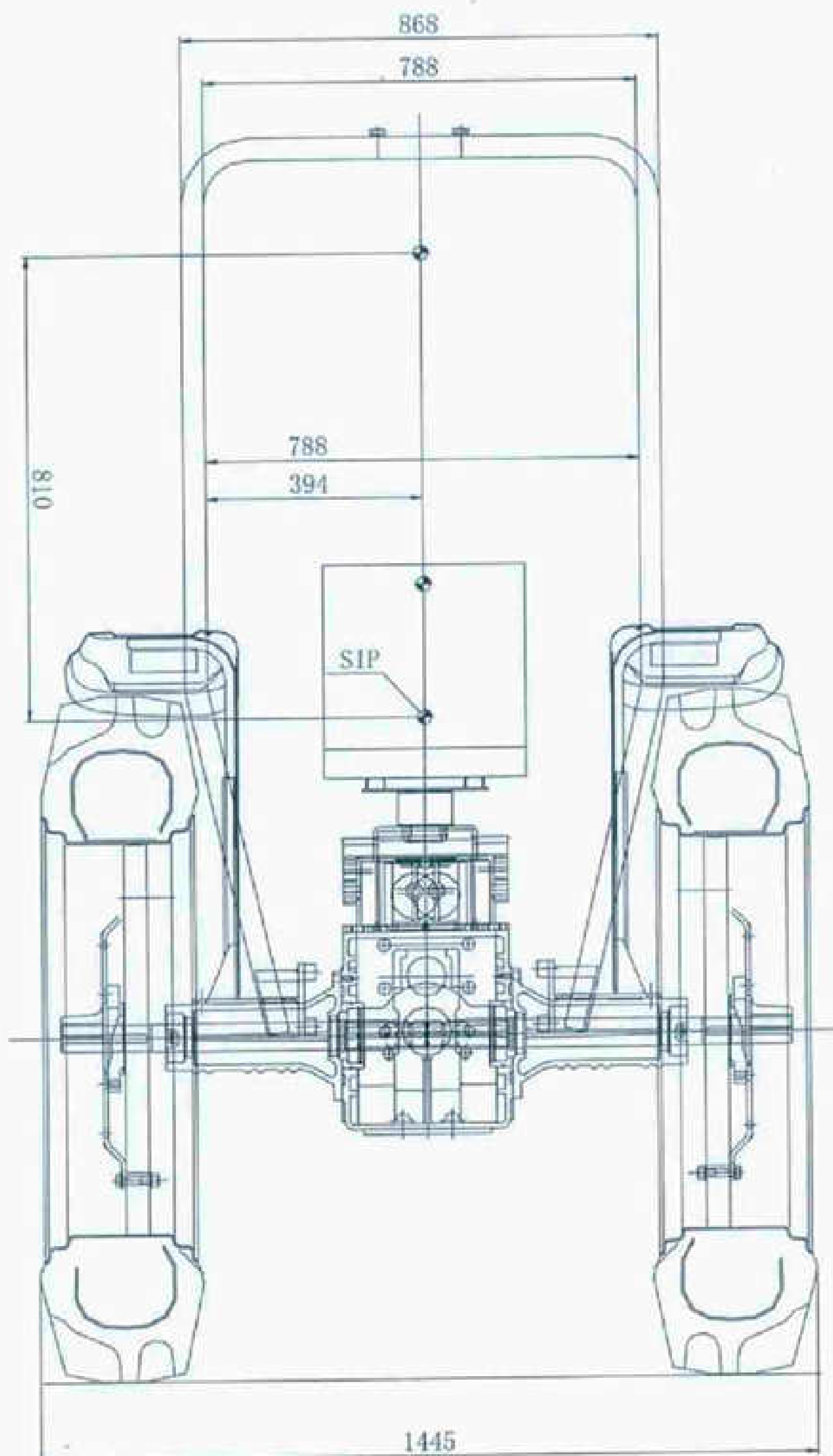
图4-2 防翻架安装于整车的结构后视图
