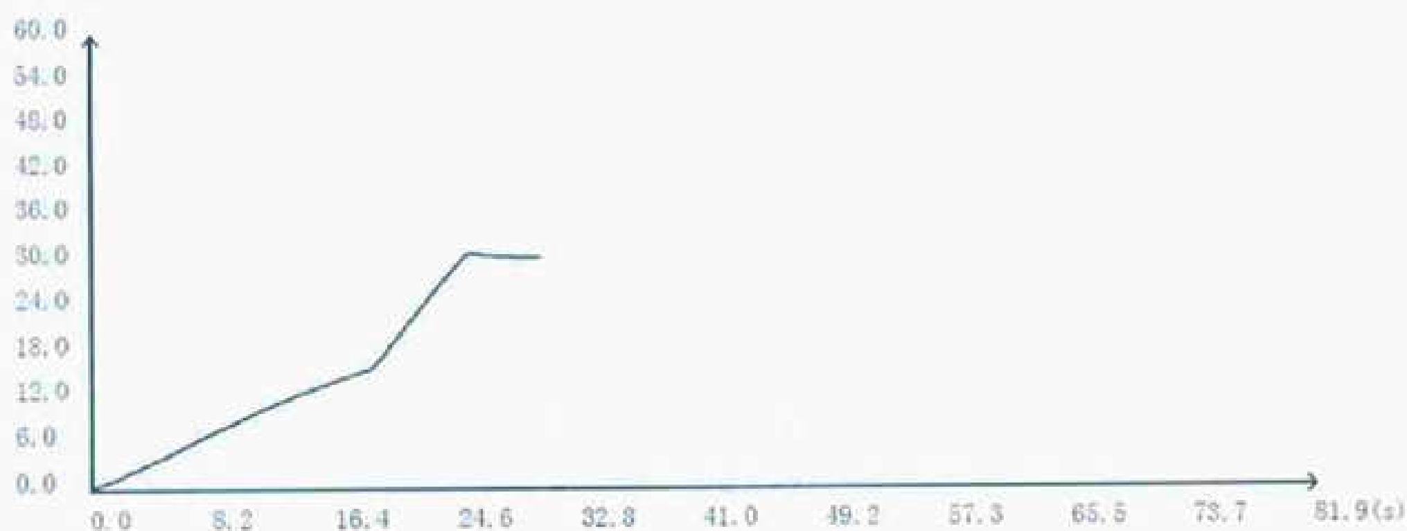
图6 后压垮试验时载荷—时间曲线图
