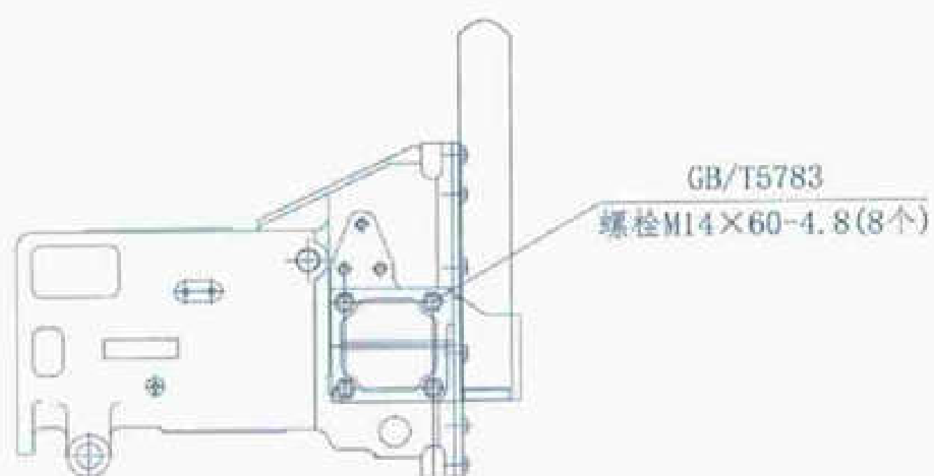
图4-4 防翻架与离合器壳体连接局部放大图
