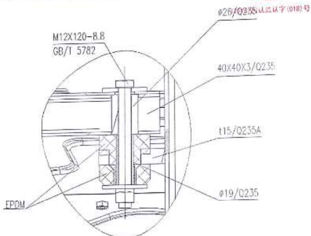
图4-10 地板连接局部剖视图 (Q-Q视图)
