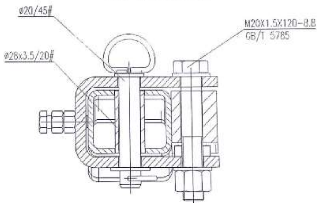
图 4-6 防翻架地板结构图
