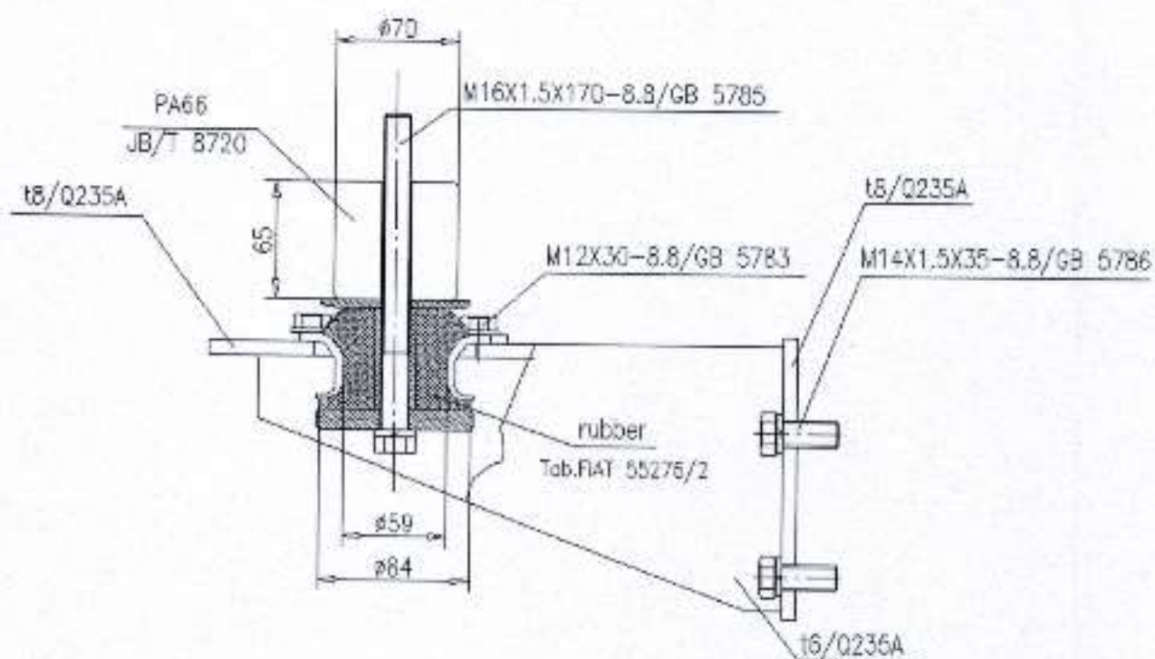
图 4-6 C-C 截面图
