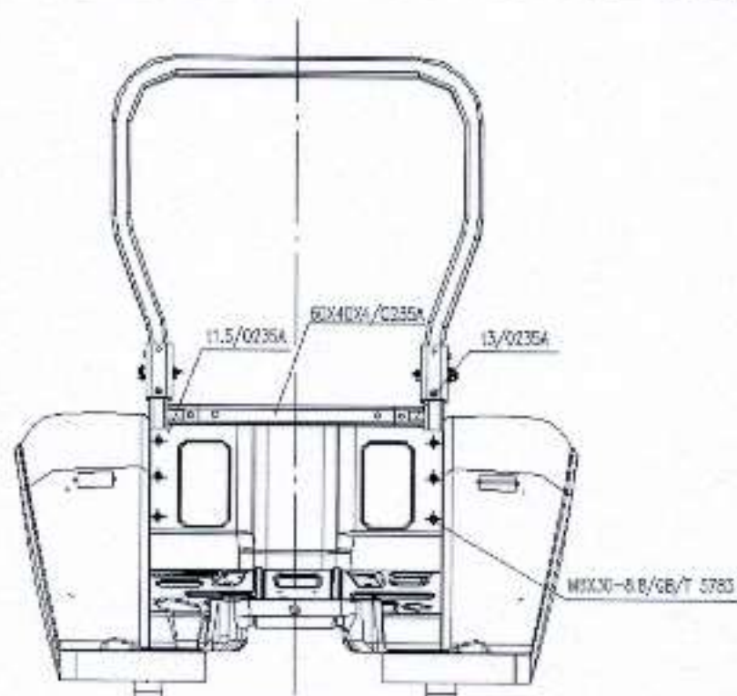
图 4-3 防撞架结构前视图
