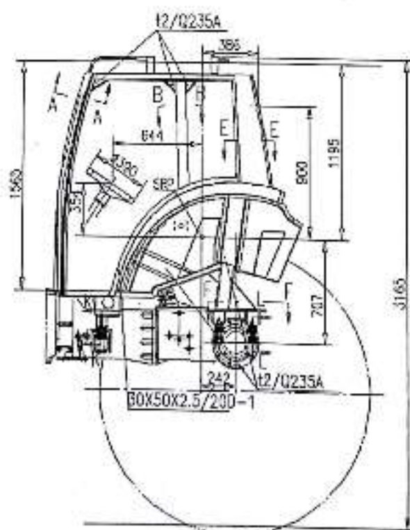
图 4-1 驾驶室结构侧视图
