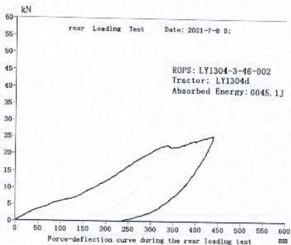
图5 后加载试验时载荷一位移曲线图
