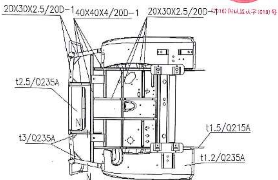
图 4-4 驾驶室地板结构图
