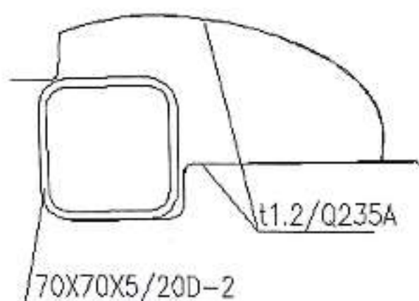
图 4-9 驾驶室侧视图中 E-E 截面图
