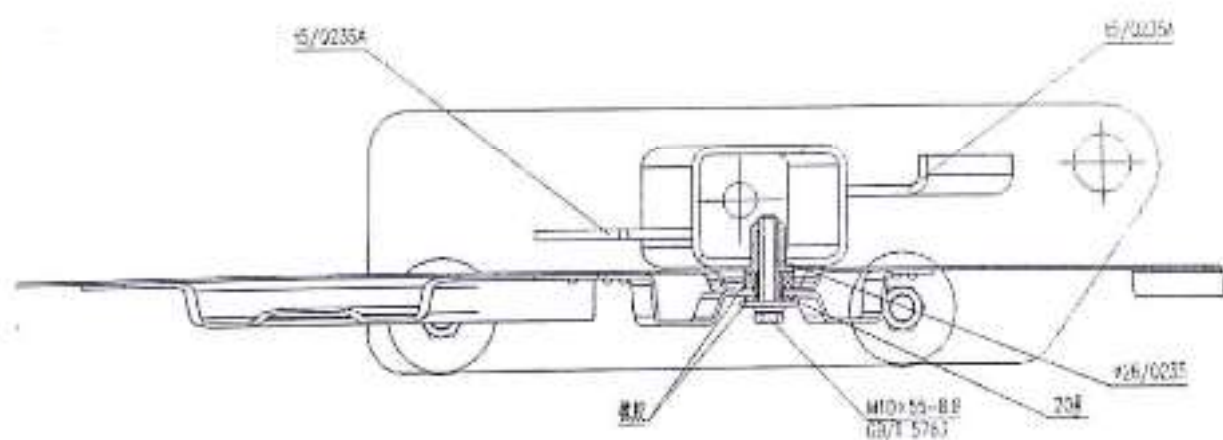
图 4-5 防翻架根部剖视图 (P-P 视图)
