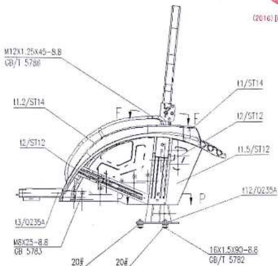
图 4-2 防翻架结构侧视图
