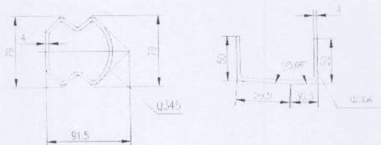
图 4-7 前、后立柱和中心柱截面图
