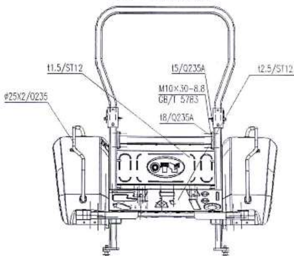
图 4-3 防翻架结构前视图
