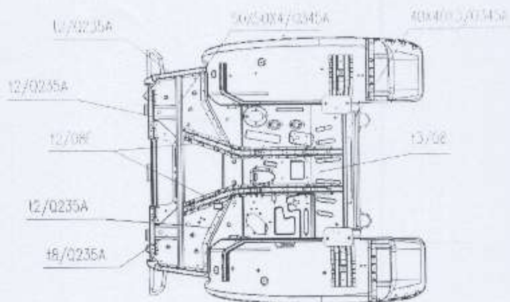
图 4-5 地板结构俯视图
