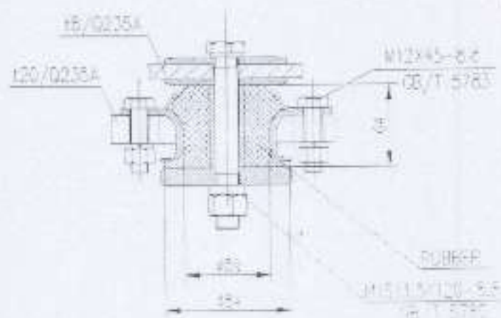
图 4-8 前支架处 G-G 剖视图
