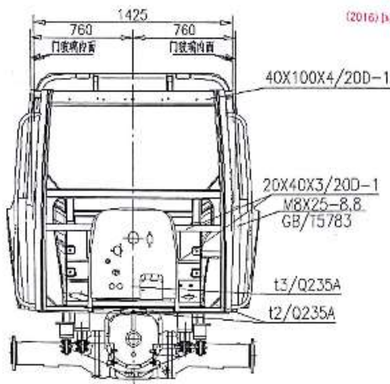
图 4-2 驾驶室结构前视图
