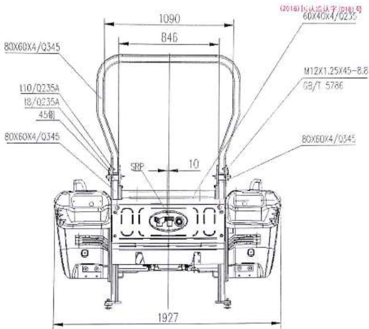
图4-4 防翻架结构后视图
