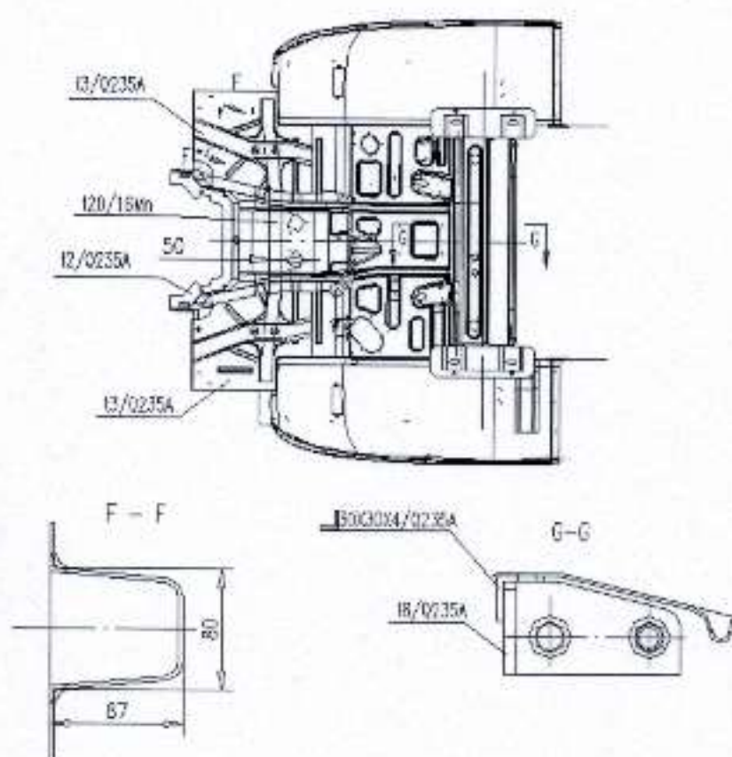
图 4-4 地板结构图
