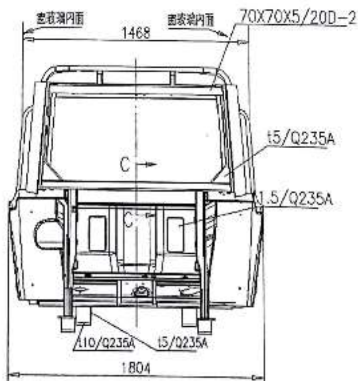
图 4-3 驾驶室结构后视图
