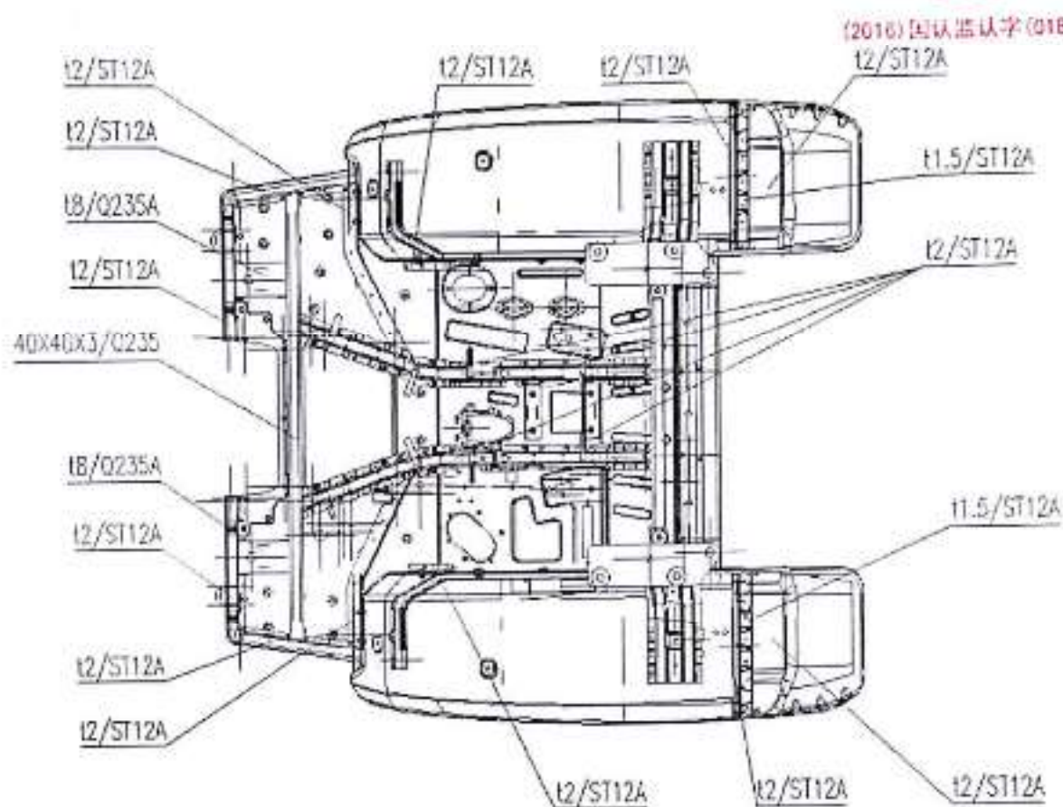
图 4-6 防翻架地板结构图
