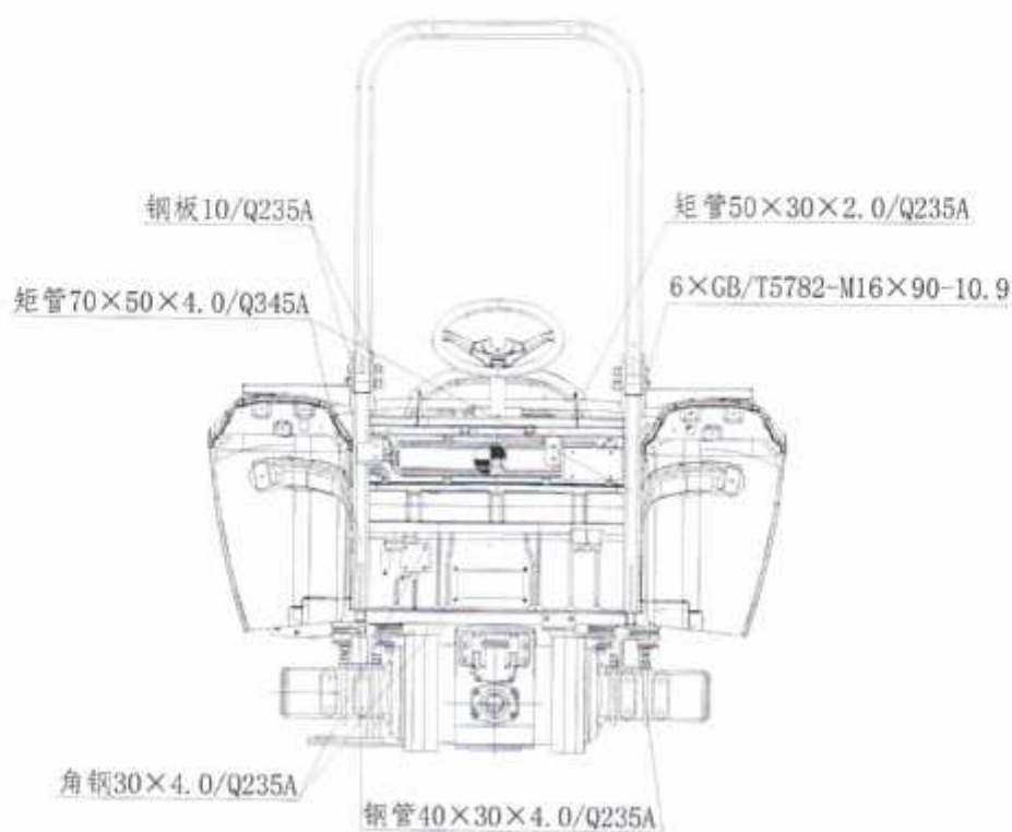
图4-7 防翻架结构后视图
