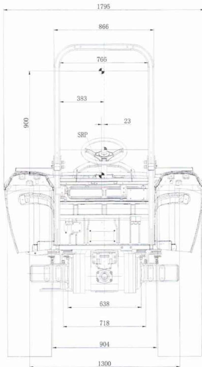
图4-2 防翻架安装于整车的结构后视图
