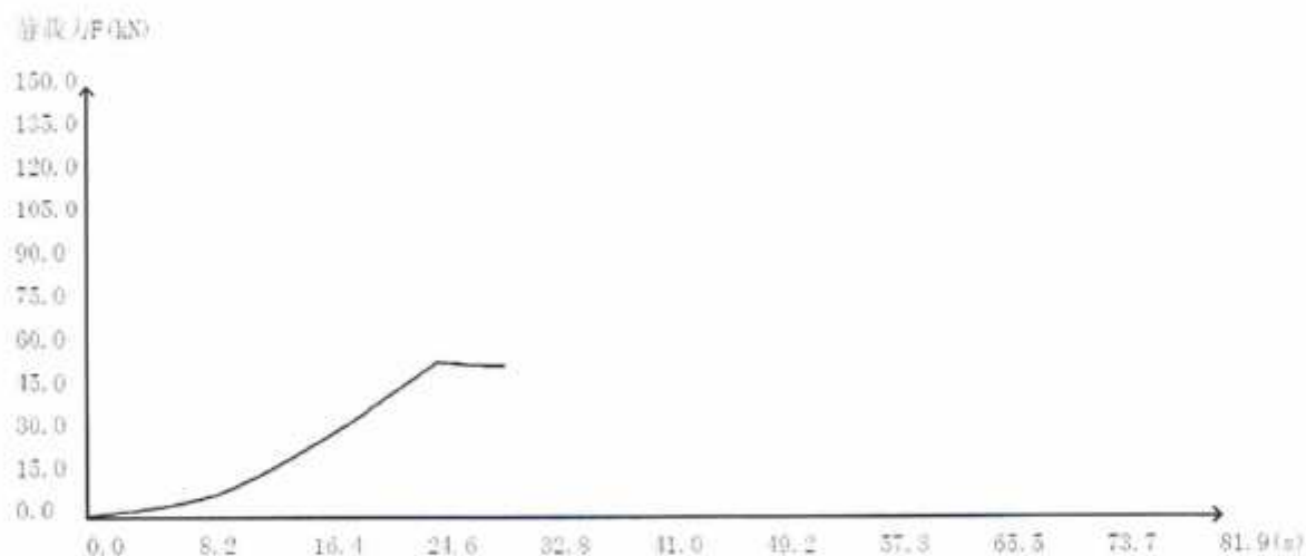
图6 第一次压垮试验时载荷—时间曲线图
