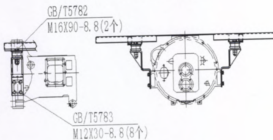
图 4-5: 防翻架前支架与箱体连接结构图
