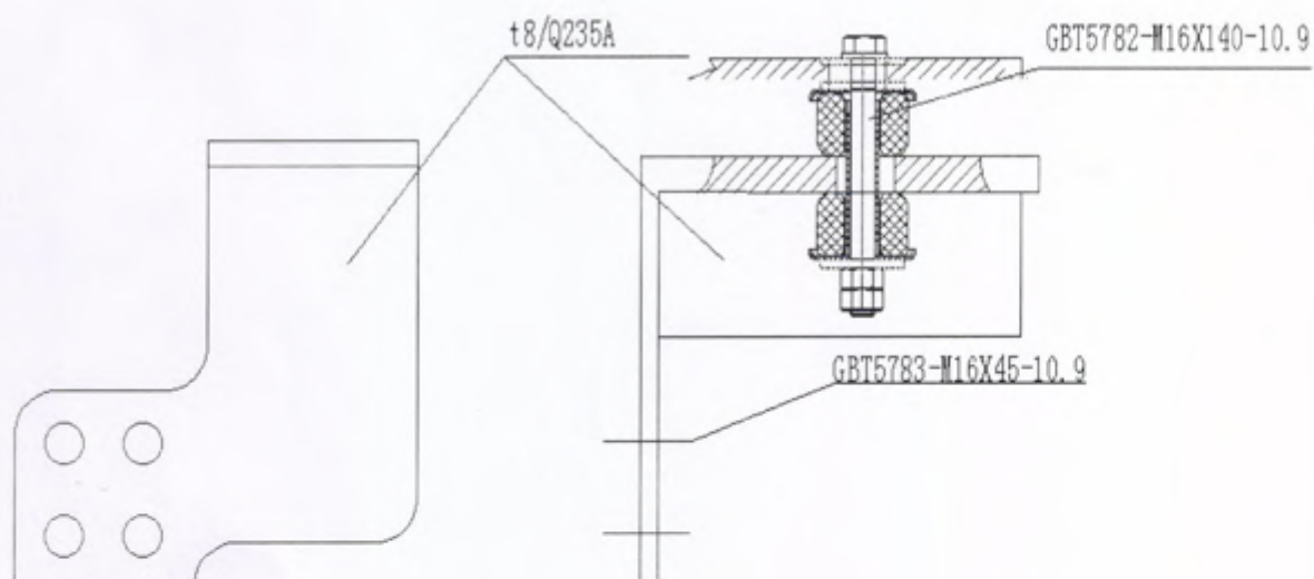
图 4-5: 驾驶室前支架结构图
