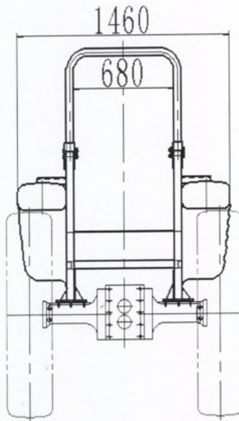
图 4-2: 防翻架整机结构后视图
