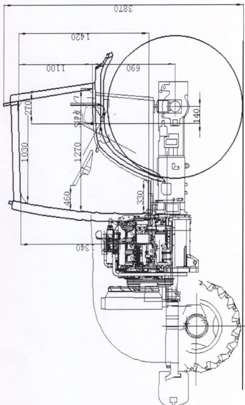
图 4-1: 驾驶室结构侧视图
