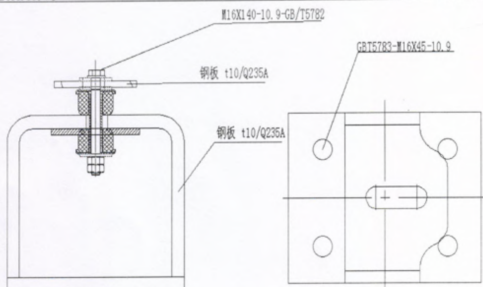
图 4-6: 驾驶室后支架结构图
