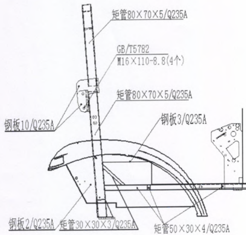
图 4-3: 防翻架侧视图
