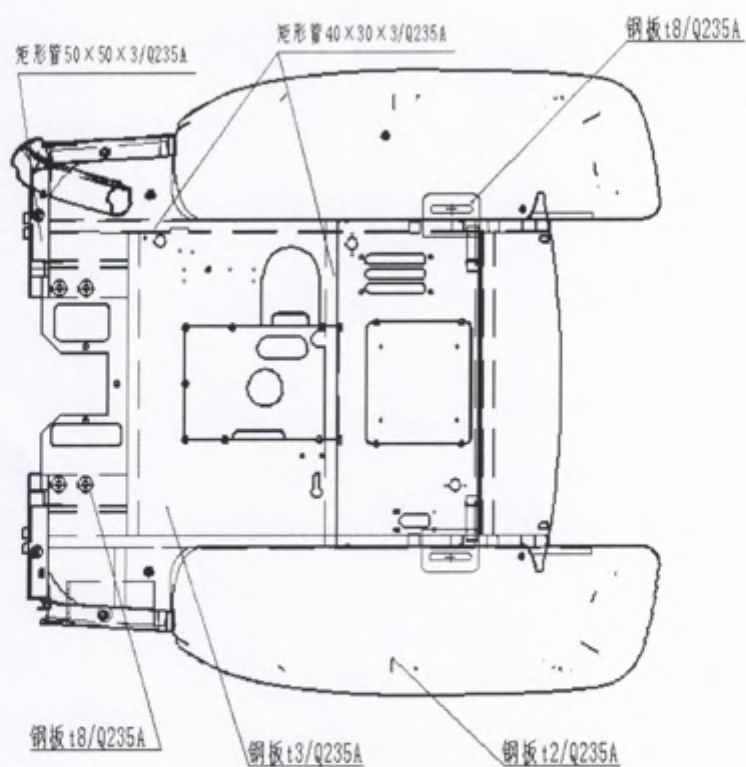
图 4-3: 驾驶室地板结构图
