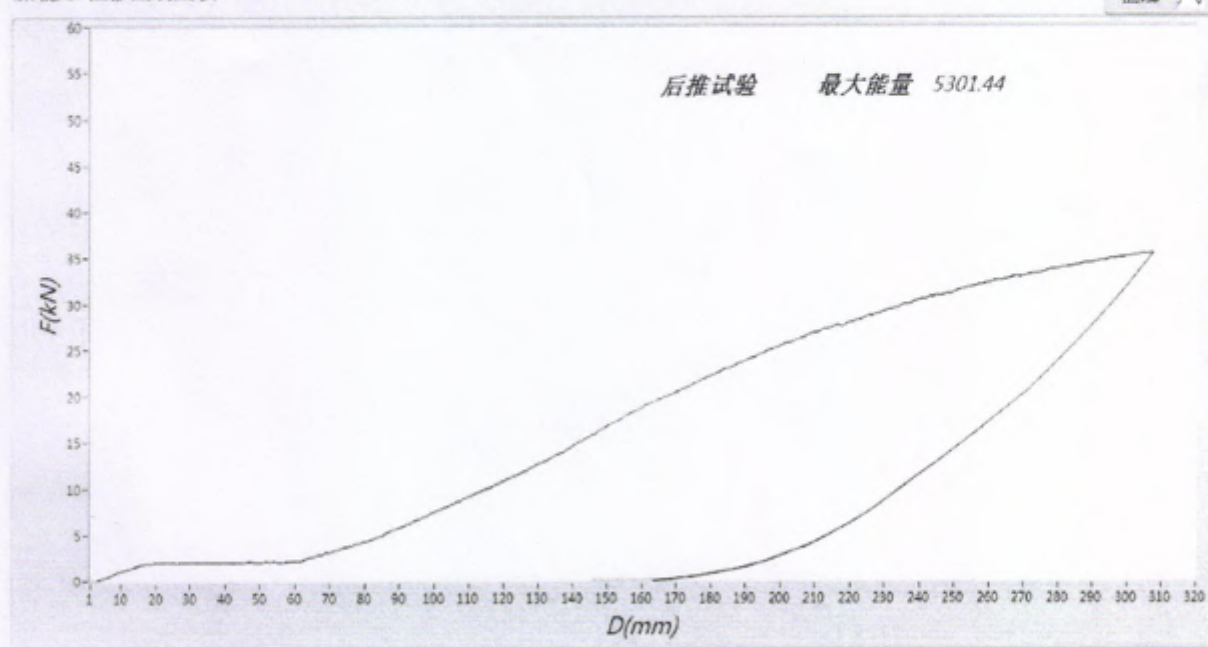
图 5: 防翻架后加载试验时载荷-位移曲线
