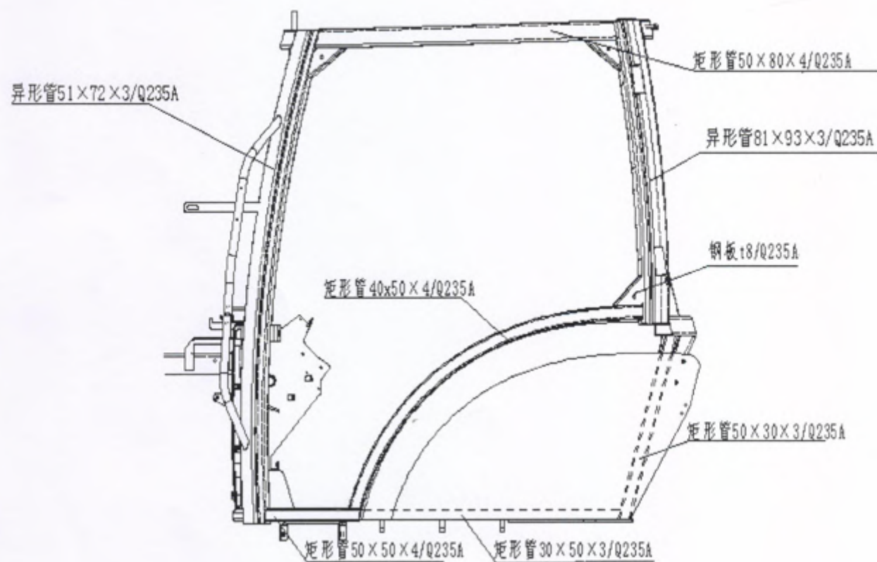
图 4-4: 驾驶室结构后视图
