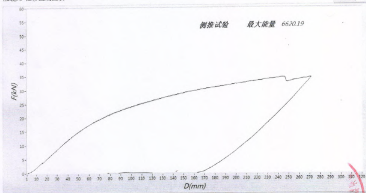
图 6: 防翻架侧加载试验时载荷-位移曲线
