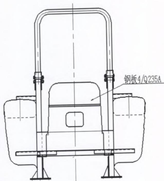
图 4-4: 防翻架结构前视图
