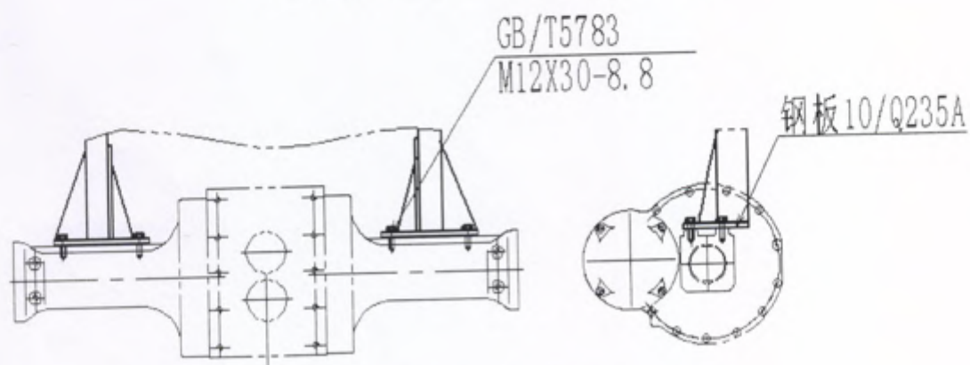
图 4-6: 防翻架后支架与后桥连接结构图
