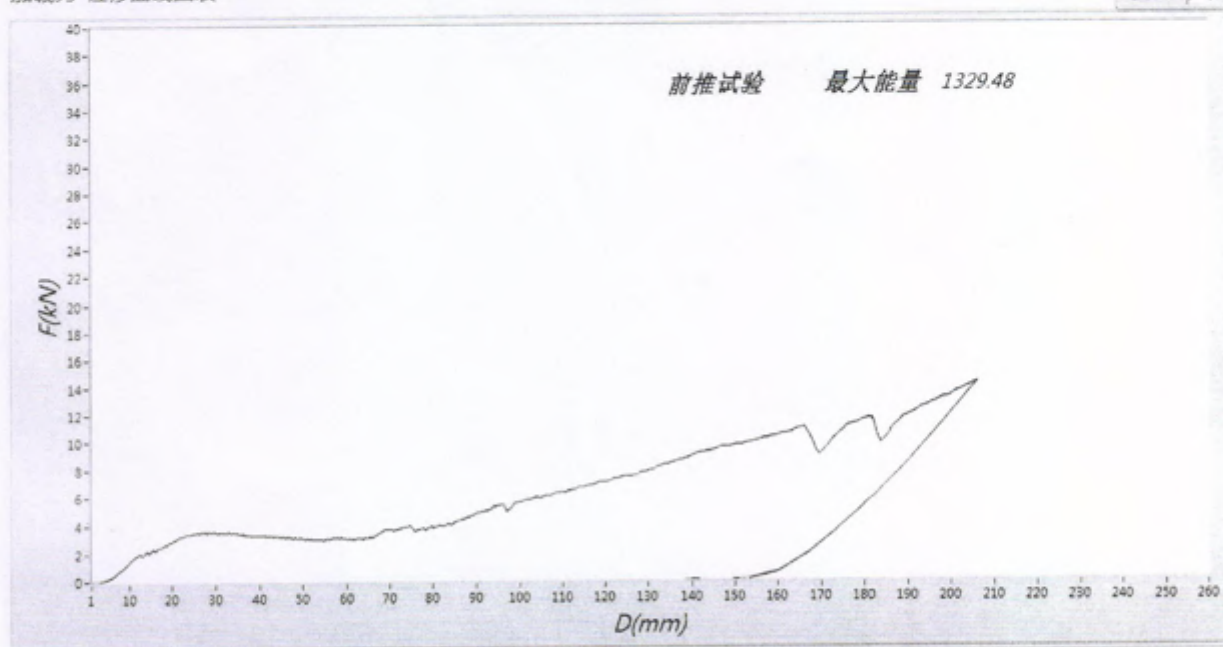
加载力-位移曲线图表
