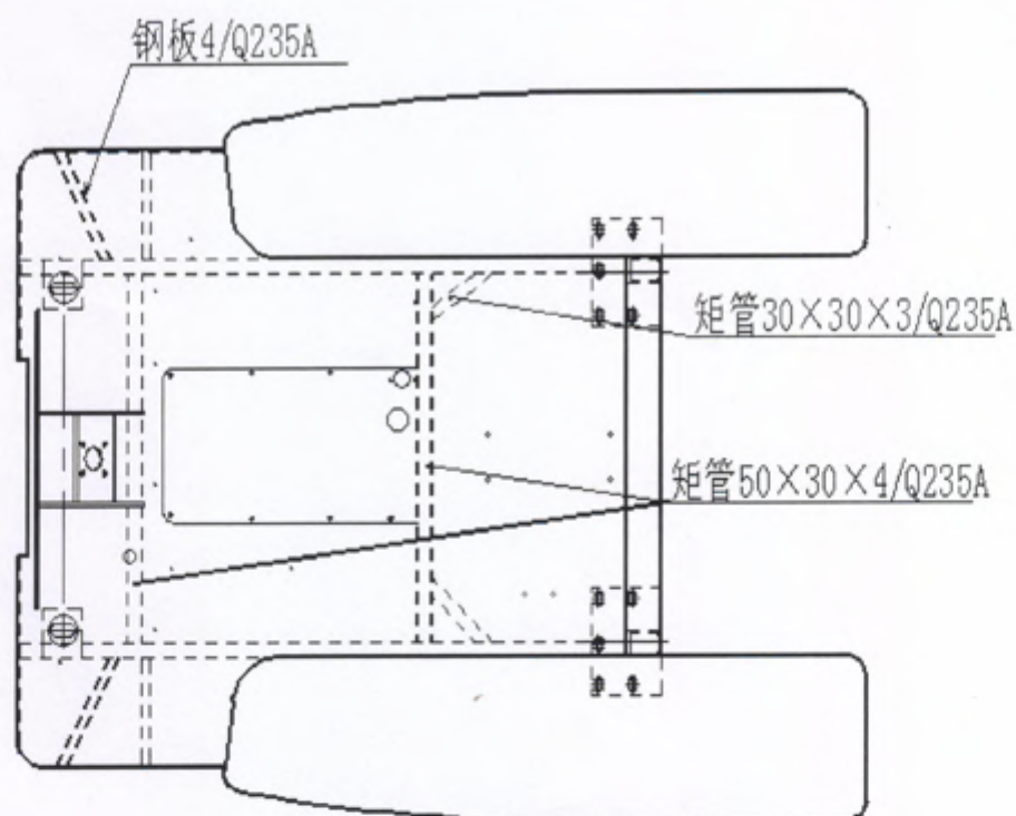
图 4-7: 防翻架底板结构图
