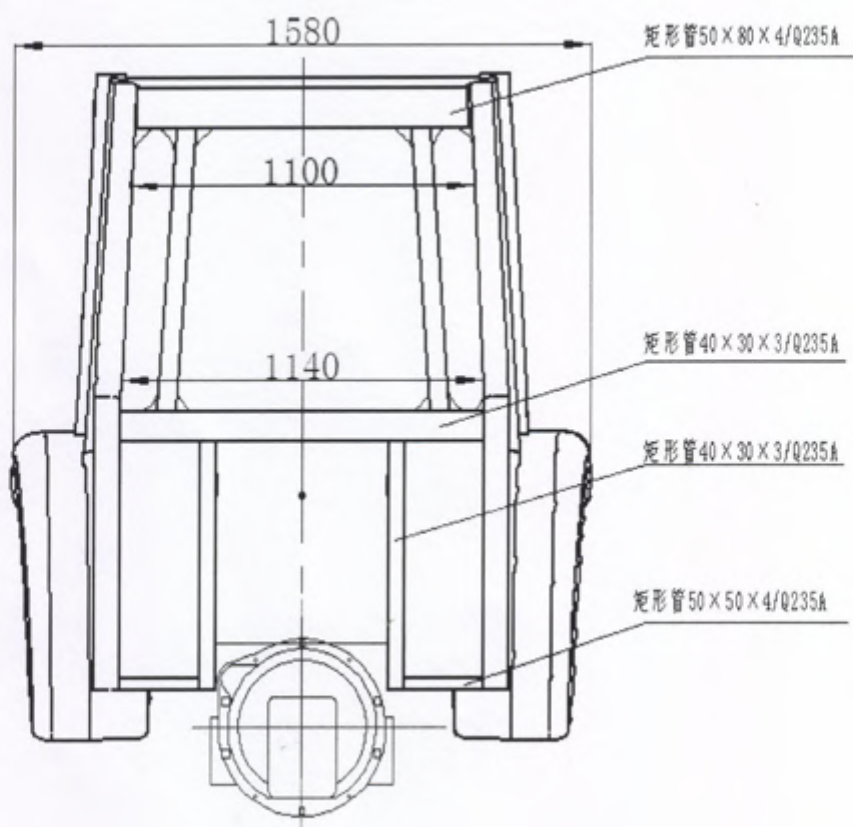
图 4-2: 驾驶室结构前视图
