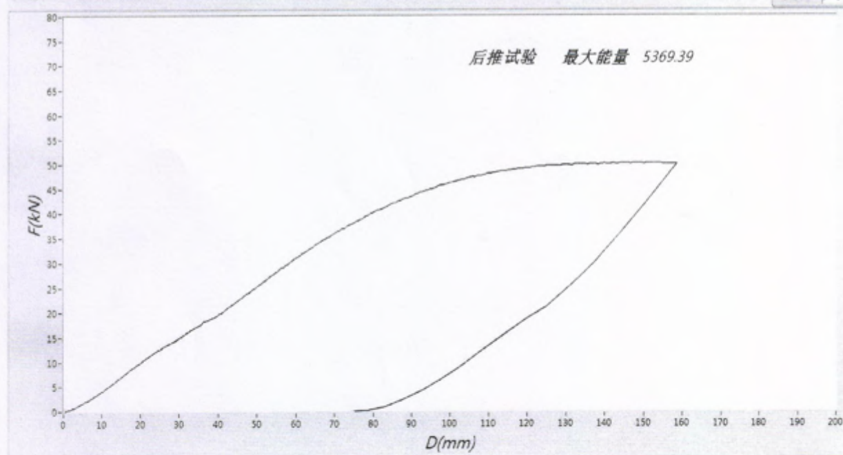
加载力-位移曲线图表
