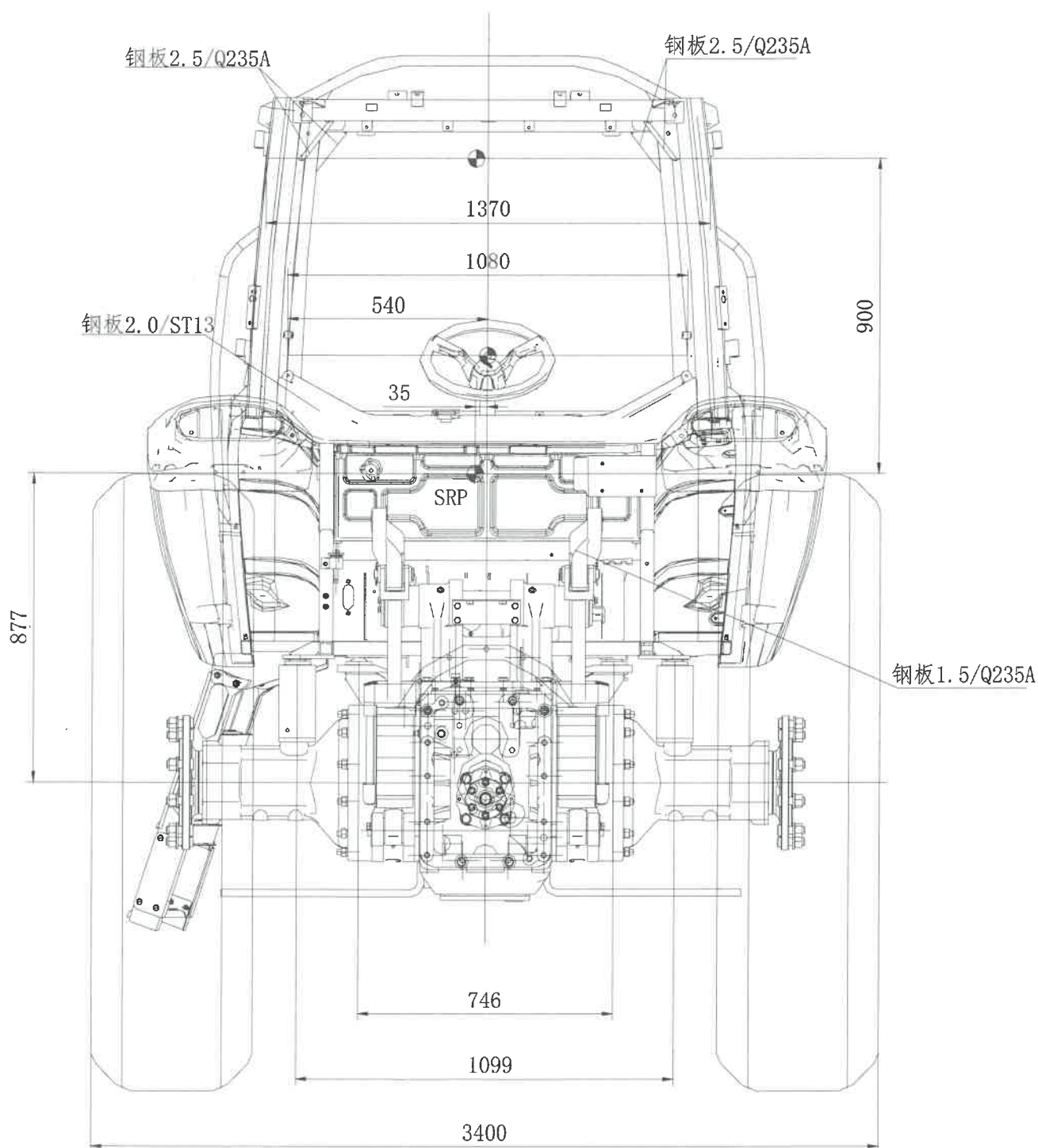
图4-2 驾驶室安装于整车的结构后视图
