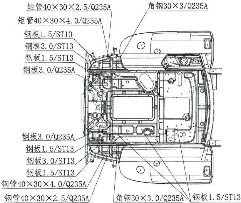
图4-5 防翻架座箱底板结构图
