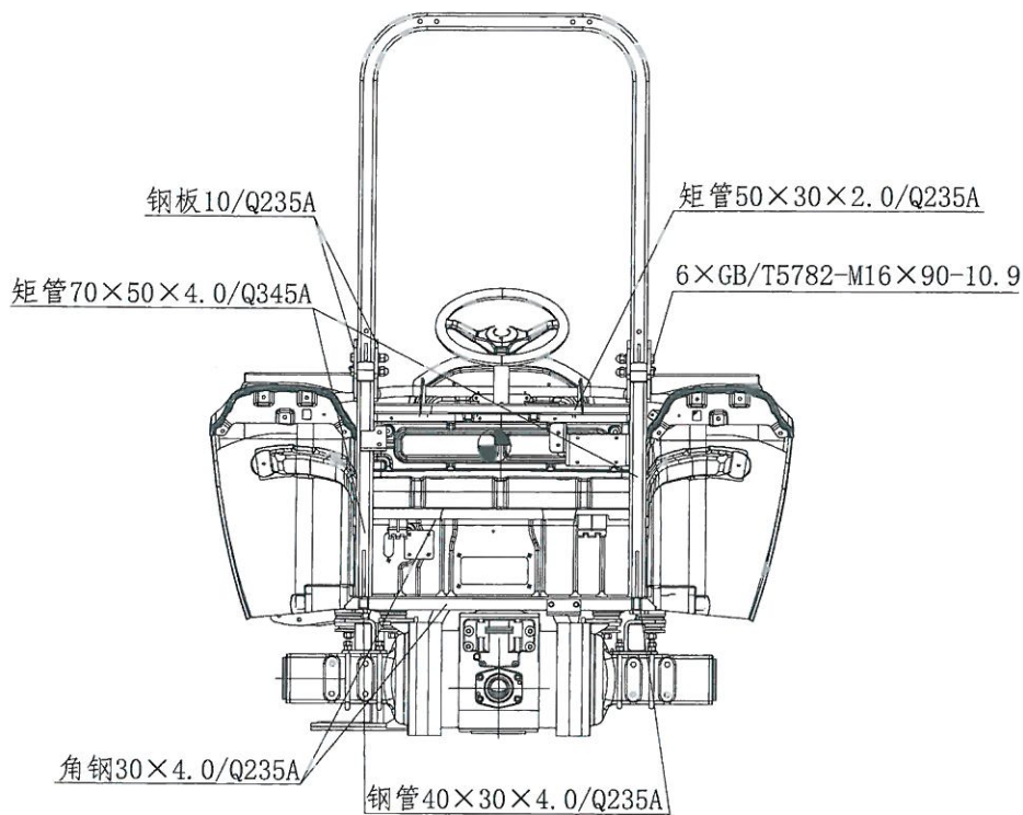
图4-7 防翻架结构后视图
