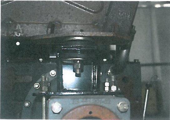
图 2 防翻架左侧安装于后桥壳体的形式 (侧 视)
