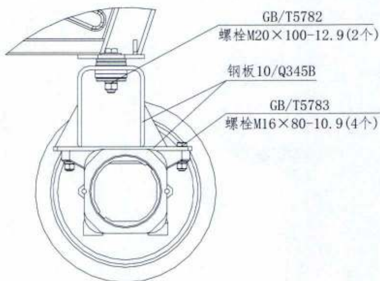
图4-6 防翻架后部安装局部放大图
