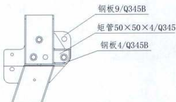
图4-5 防翻架折叠处连接板结构图
