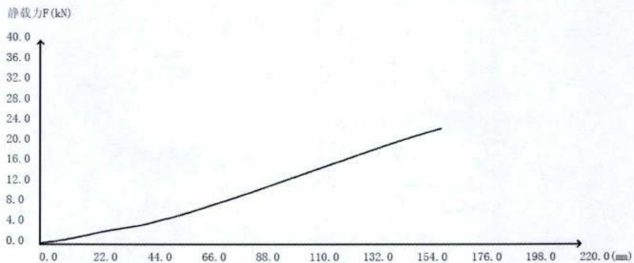
图9 第二次纵向(左前侧)试验时载荷—位移曲线图
