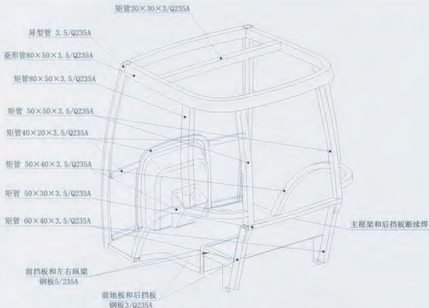
图4-4 驾驶室结构图
