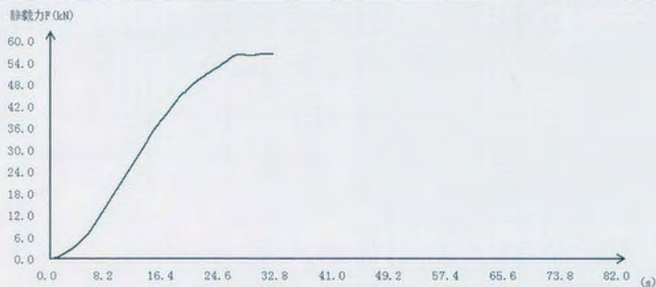
图8 第二次压垮试验时载荷—时间曲线图
