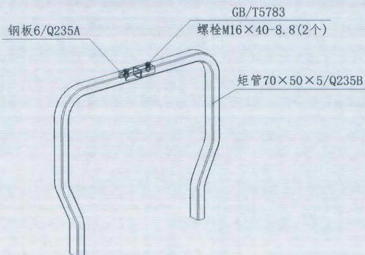
图4-4 防翻架结构图
