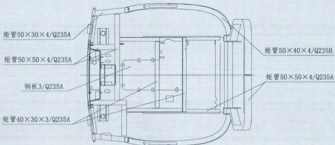
图4-3 防翻架底部结构图
