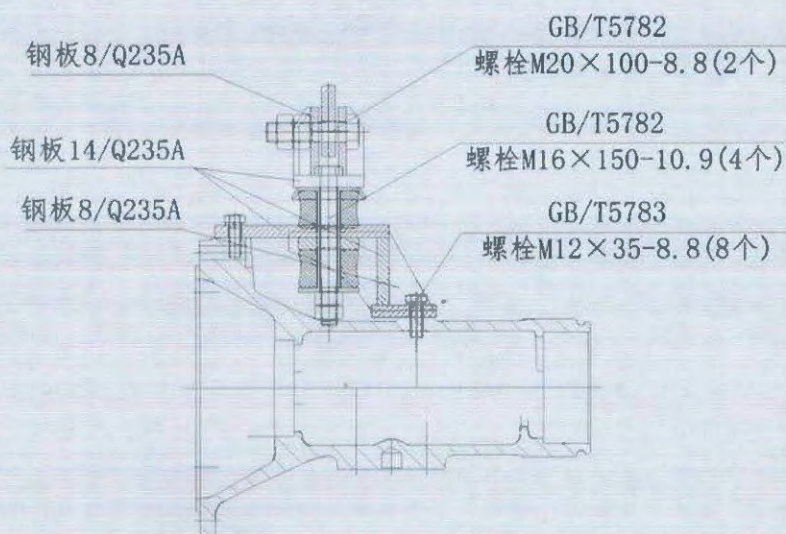
图4-6 防翻架后部安装局部放大图
