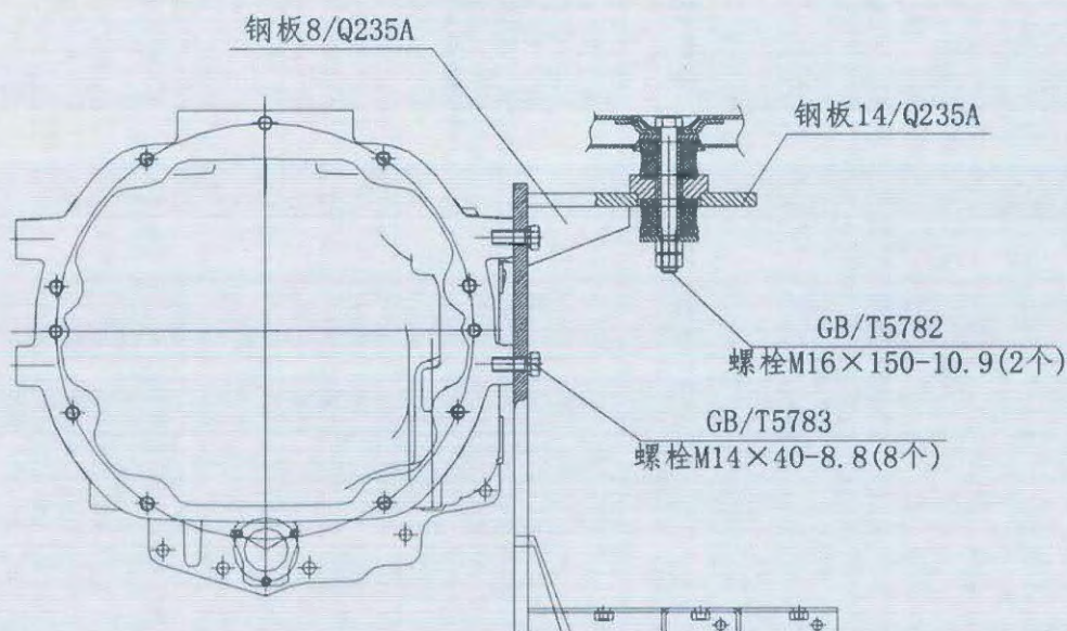
图4-5 前部安装局部放大图
