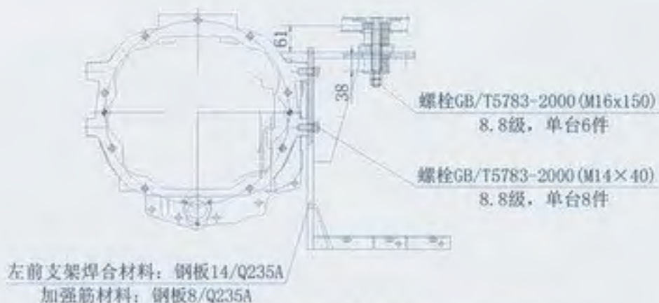
图4-5 驾驶室前部与变速箱壳体连接局部放大图
