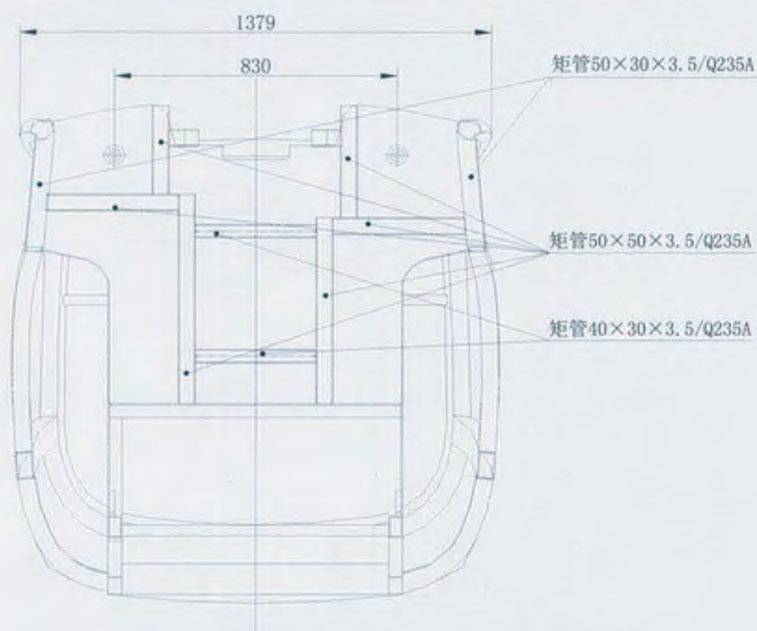
图4-6 驾驶室结构俯视图
