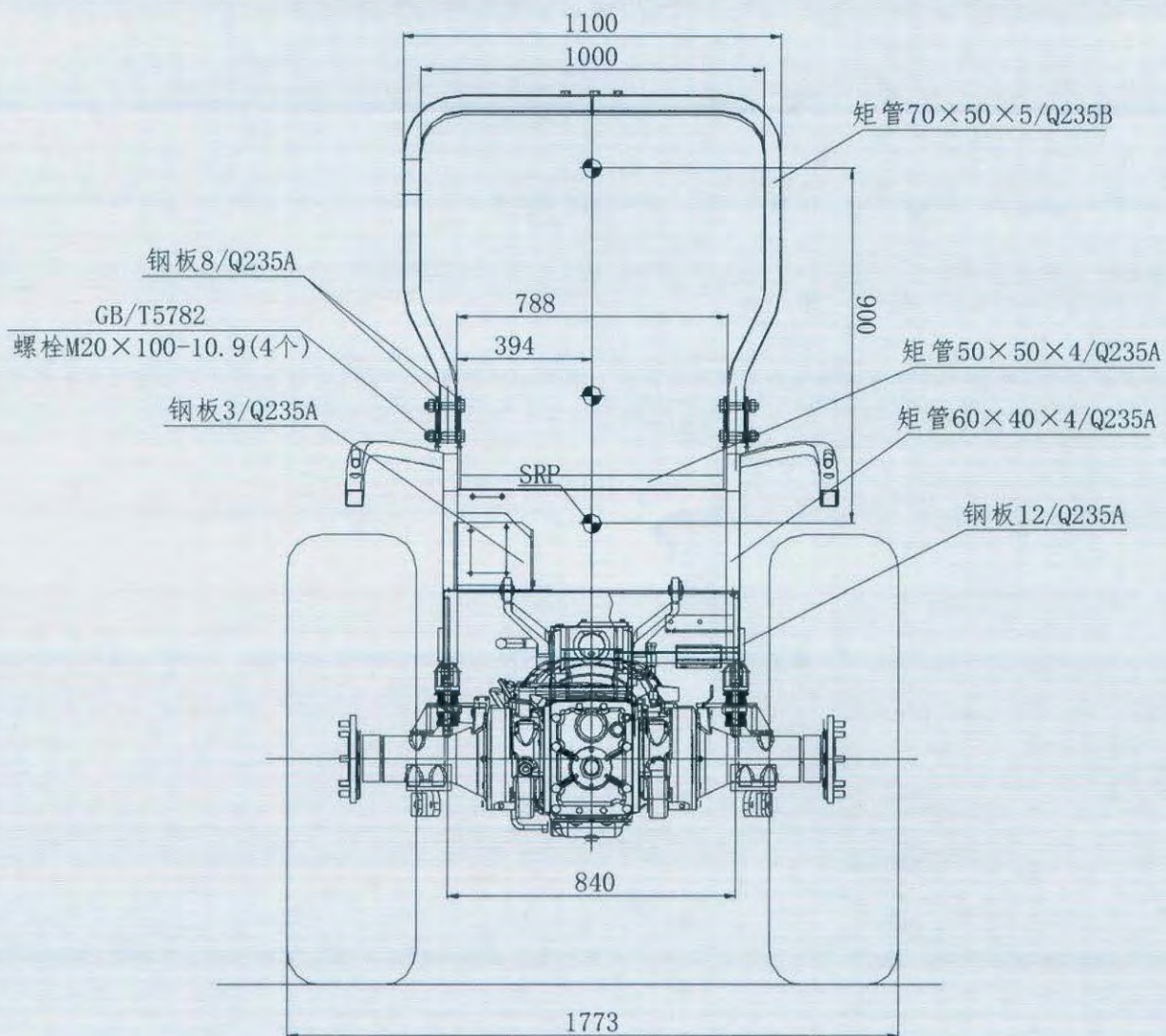
图4-2 防翻架安装于整车的结构后视图
