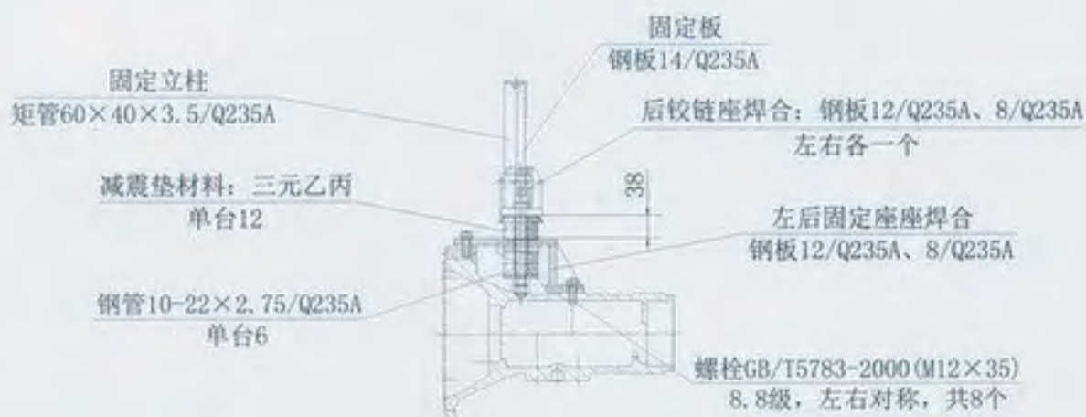
图4-3 驾驶室后部与后轴壳体连接局部放大图
