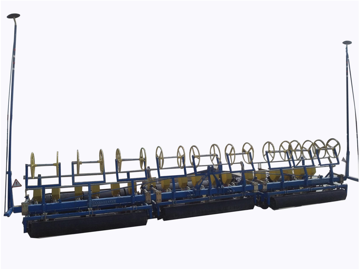
2MBJ-3/18 型机械式精量铺膜播种机
