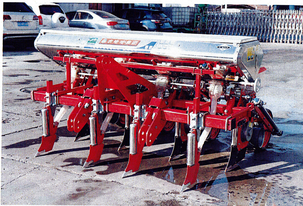
2BYFSF-4 型玉米免耕施肥精播机
