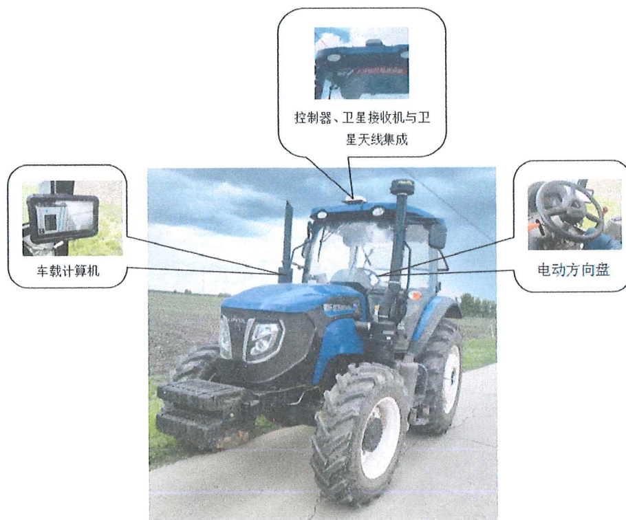
AG12BD-2.5GD 型农业机械导航及自动作业系统
