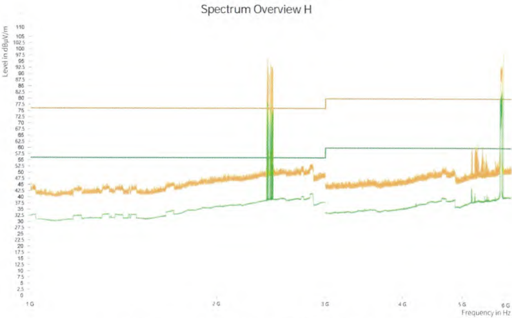
1GHz~6GHz 辐射骚扰测试结果图（水平极化）
