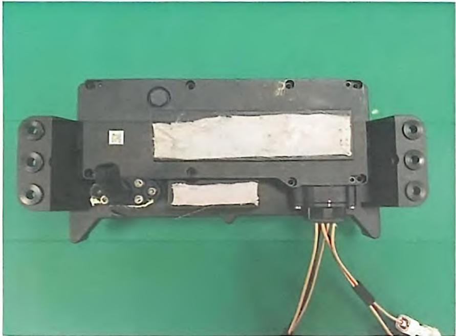
北斗飞行控制系统 背面图
