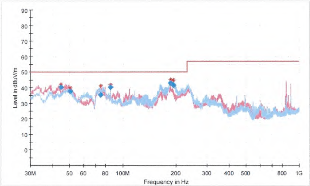
30MHz~1000MHz 辐射骚扰测试结果图
